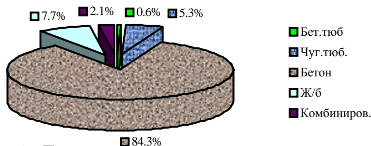
Рисунок 1. - Процентное соотношение видов крепи, распространенных в вертикальных стволах Донбасса
